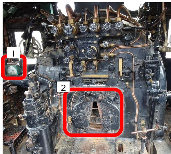
1 速度計 2 石炭を投げ込むところ
